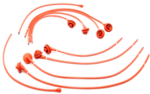
ZK0504 Zündkabelsatz | Ignition Lead Set Ferrari
