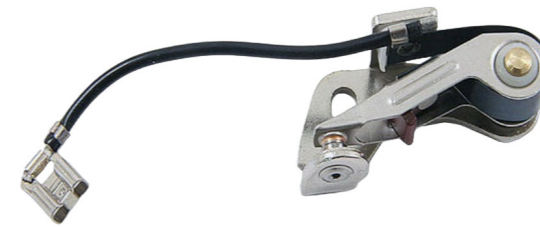
CS0414 Zündkontakt | Breaker Point gemäß 1 237 013 142 according to 1 237 013 142 Mercedes-Benz
