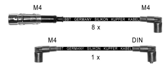
ZK0416 Zündkabelsatz | Ignition Lead Set Mercedes Benz
