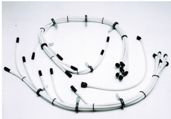
ZK0506 Zündkabelsatz | Ignition Lead Set Ferrari
