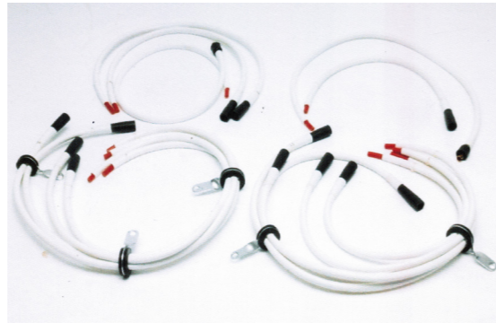
ZK0503 Zündkabelsatz | Ignition Lead Set Ferrari
