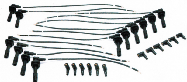
ZK0513 Zündkabelsatz | Ignition Lead Set Ferrari
