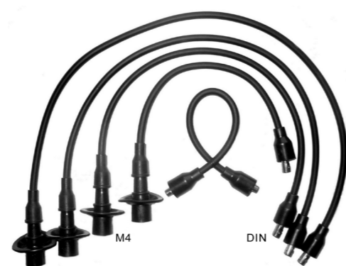
ZK0215 Zündkabelsatz | Ignition Lead Set Porsche
