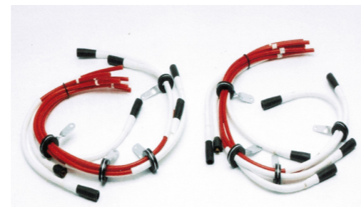
ZK0511 Zündkabelsatz | Ignition Lead Set Ferrari
