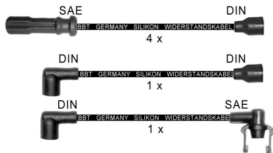
ZK0151 Zündkabelsatz | Ignition Lead Set Volvo
