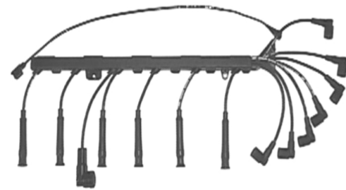
ZK0922i Zündkabelsatz | Ignition Lead Set BMW
