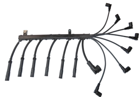
ZK0944 Zündkabelsatz | Ignition Lead Set BMW
